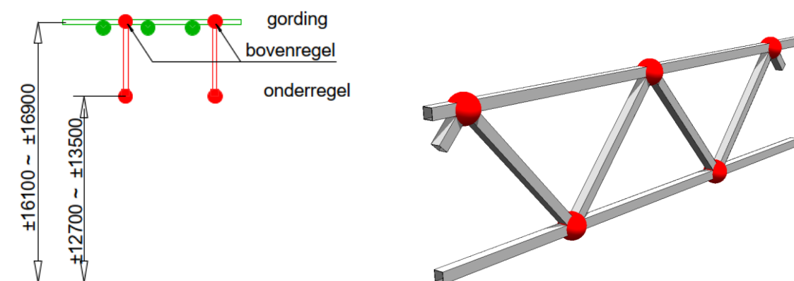
figuur 10: Ophangpunten Westhal
