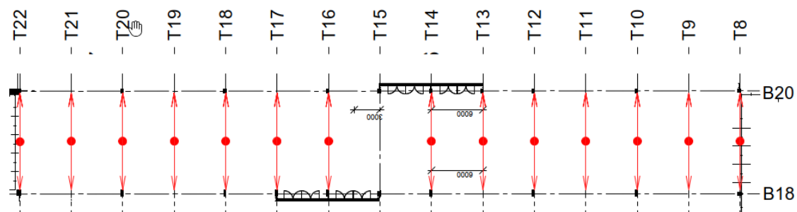
figuur 15: Ophangpunten aan stalen liggers (●)
